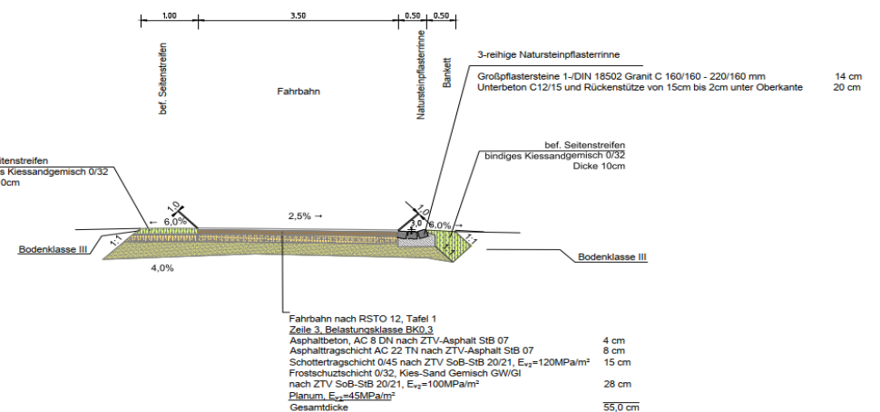
Schnitt A - A von St. 0 + 022,30 bis St. 0 + 329,15
