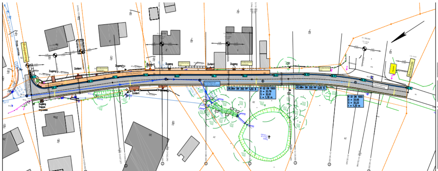
Auszug Lageplan
