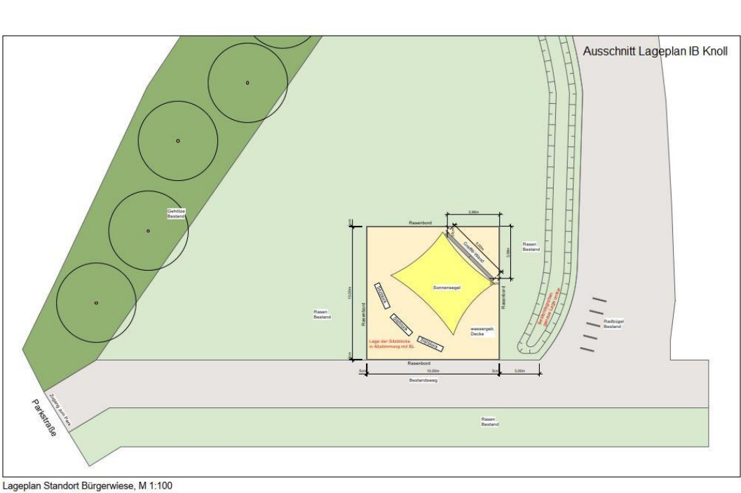
Lageplan Standort Bürgerwiese, M 1:100
