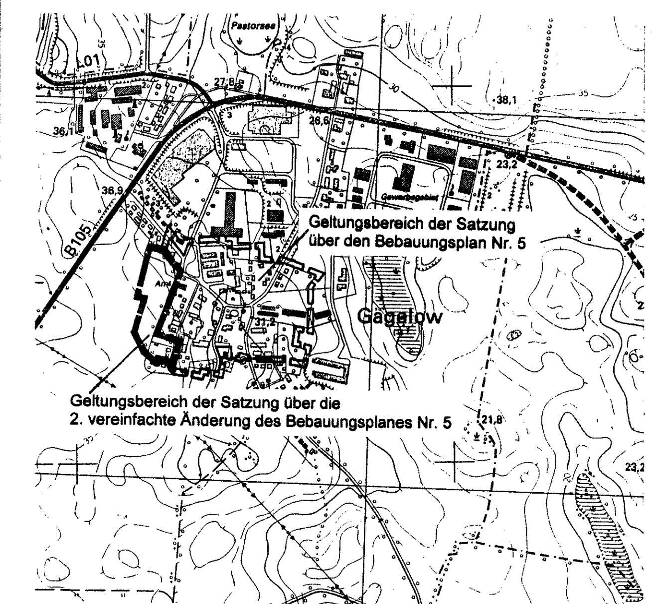
Übersichtsplan M 1:10000
